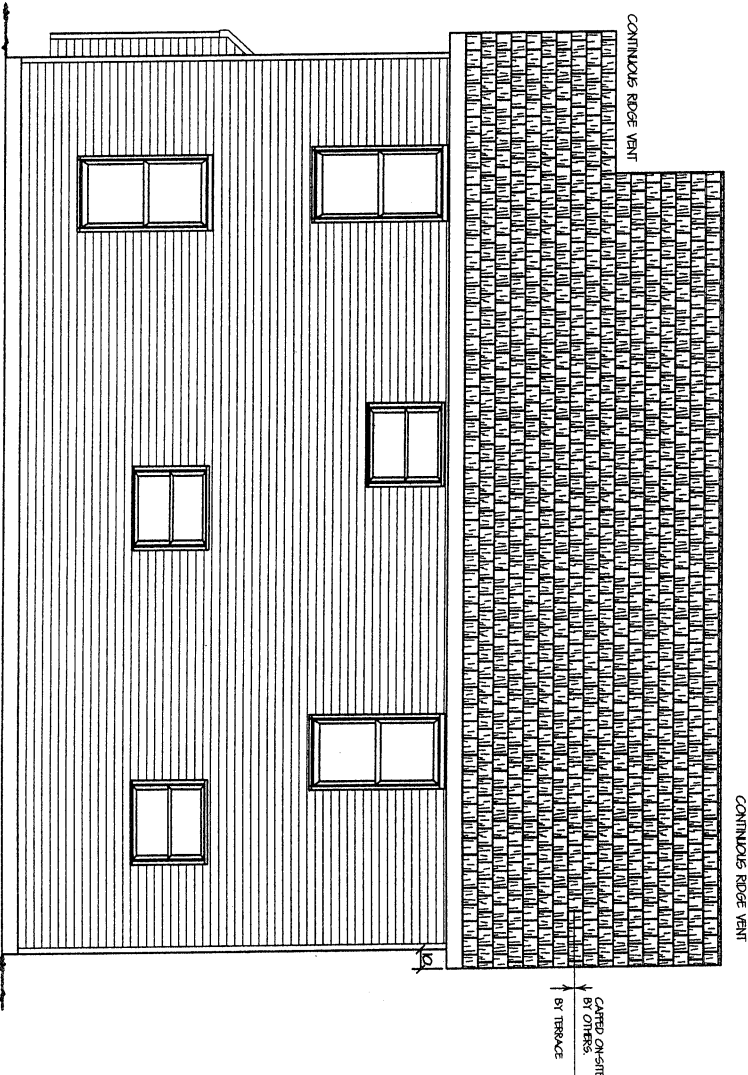
RIGHT ELEVATION
